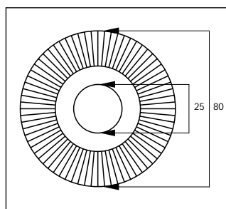
Cilindro poliamida
